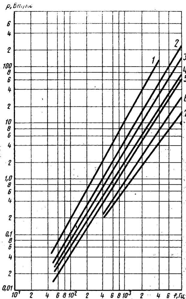
Зависимость P_{0,5} от частоты для сплавов марок:
